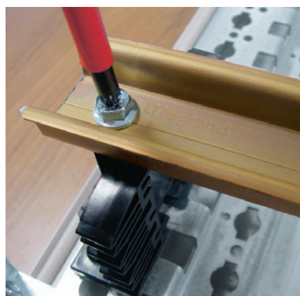
Bornier de sortie en bas d'armoire sur rail réf. 206 02.
