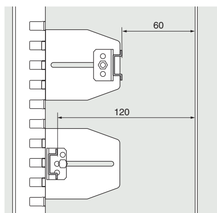
Distances minimum et maximum entre rail réf. 206 02/52 et plastron
