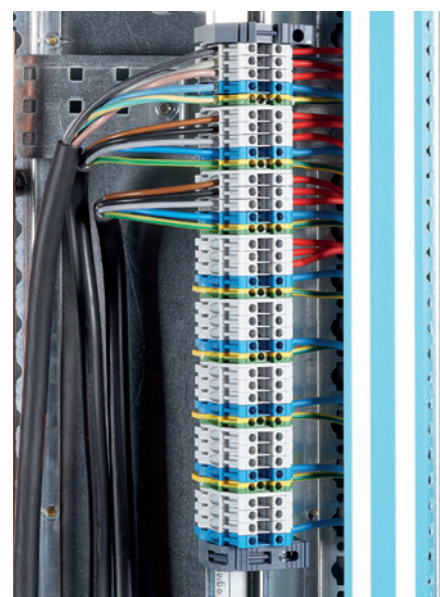
Exemple de réalisation d'un bornier vertical à l'aide du support universel pour gaines à câbles interne réf. 201 96
