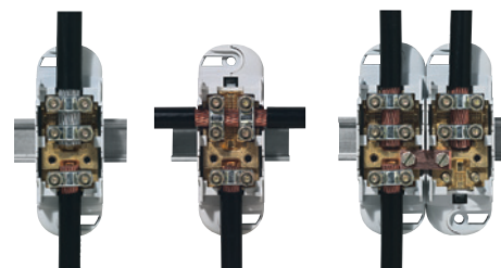
Exemples de raccordements réalisables. (avec réf. 0 374 80)
