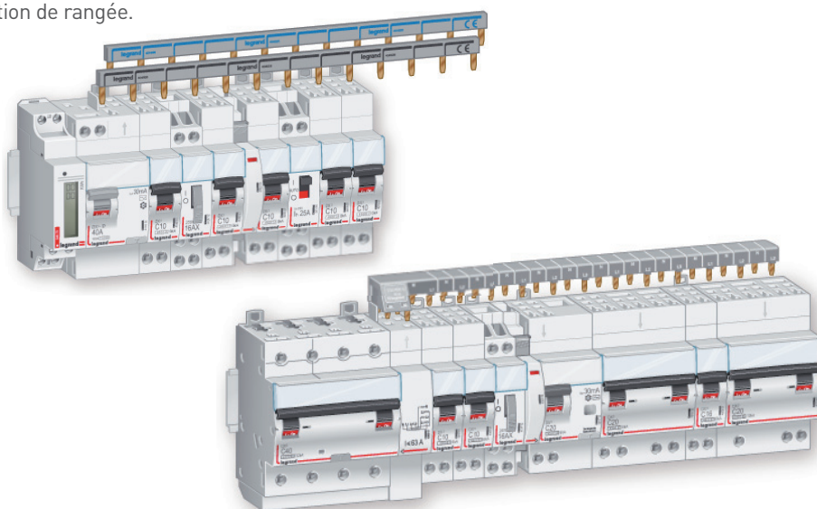
Exemples de raccordements monophasé (réf. 4 049 26) et triphasé (réf. 4 052 01)
