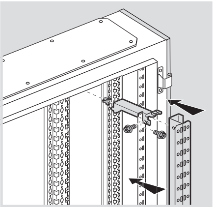
Le montage d'une gaine à câbles interne est identique aux enveloppes IP 30 (voir page 10).
