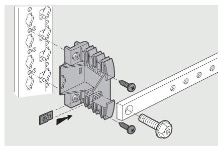
Montage sur les supports isolants réf. 0 200 90 (classe II)
