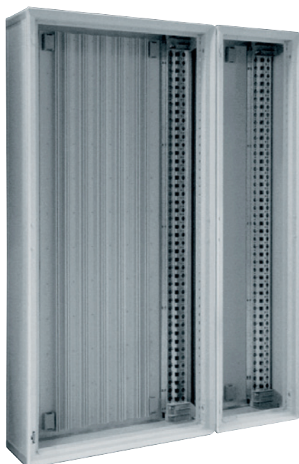
Jumelage d'un coffret et d'une gaine à câbles.
