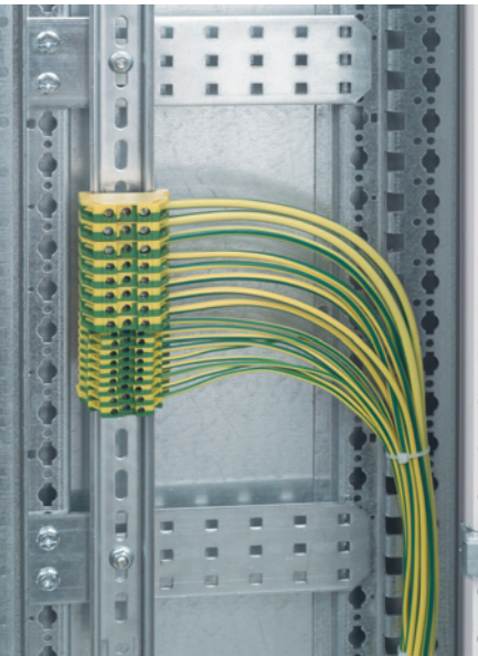
Blocs de jonction Viking sur rail à l'aide du support universel réf. 0 201 95 (pour gaines à câbles externes)
