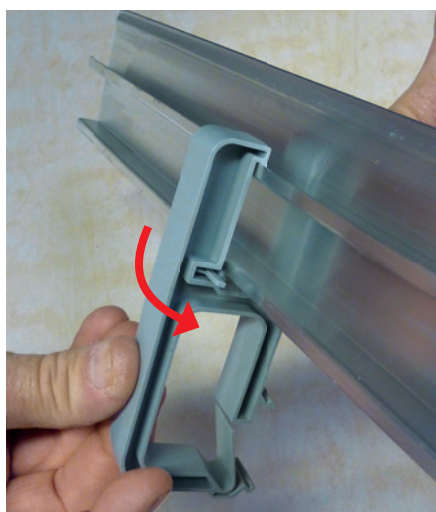
Bracelet réf. 4 052 25 pour montage sur rail alu
