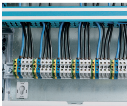
Bornier de sortie en bas d'armoire sur rail réf. 206 02.
