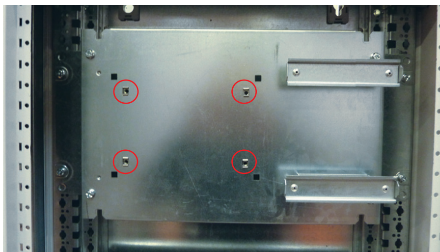
Fixation des platines réf. 4 011 81 et 4 011 91 + 4 011 93.
