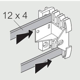
Montage sur support isolant réf. 0 200 90
