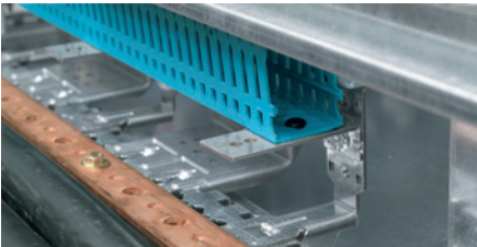
Les goulottes se fixent sur les supports à l'aide des rivets isolants livrés
