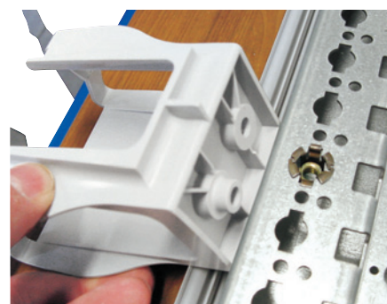
Bracelet réf. 0 200 94 - pour montage sur rail universel
