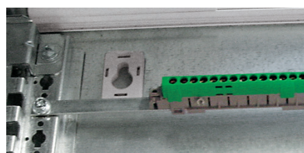
Montage direct du barreau plat sur les montants fonctionnels
