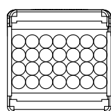
Ø 10mm Max 28 cables
