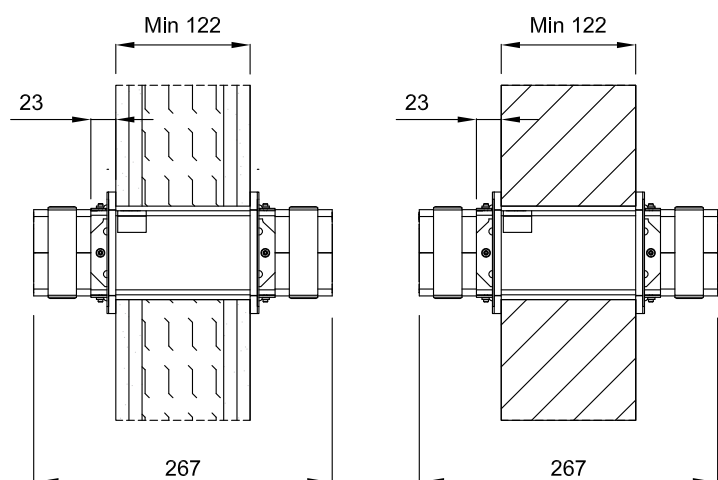
CM250120 + CM250018 (2x) EZP233WT + EZD33T (2x)
