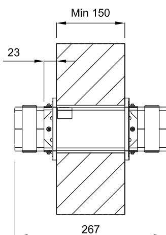
CM250120 + CM250018 (2x) EZF233WT + EZD33T (2x)
