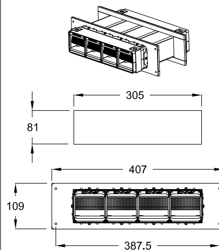
CM250140 + CM250018 (4x) EZF433WT + EZD33T (4x)
