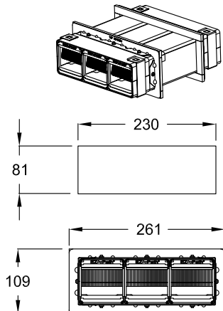
CM250130 + CM250018 (3x) EZP333WT + EZD33T (3x)
