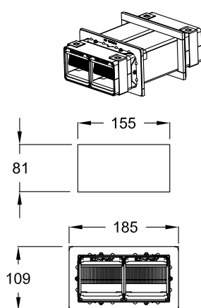
CM250120 + CM250018 (2x) EZP233WT + EZD33T (2x)
