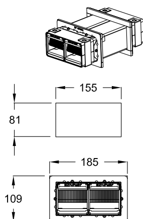
CM250120 + CM250018 (2x) EZF233WT + EZD33T (2x)
