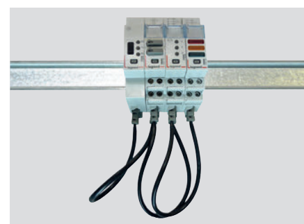
LIAISON PAR CORDON
