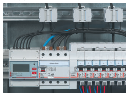
RACCORDEMENT AVEC TI
