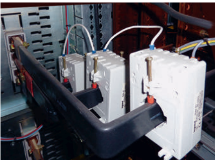
MESURE HAUTES INTENSITÉS
