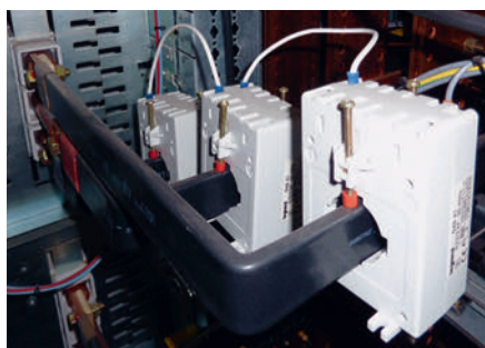
Transformateurs d'intensité montés directement sur les barres souples
