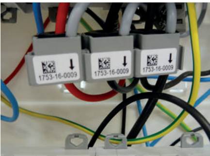
MESURE JUSQU'À 63 A
