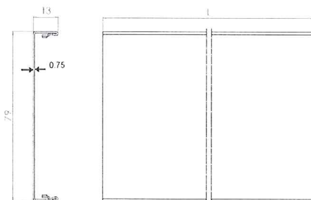
Deckel für Wandkanal GWO
