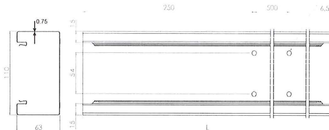
Wandkanal GWO 110x63
