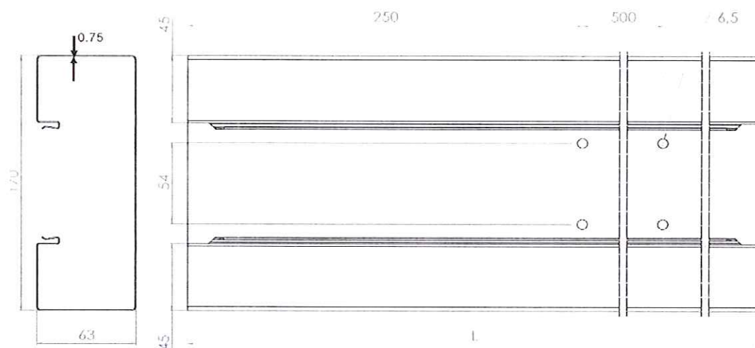
Deckel für Wandkanal GWO
