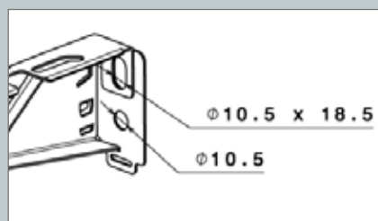
Bevestigen met 2 schroeven M10 (zie gaten)
