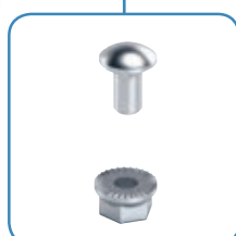
P31+ KABELGOOT BEVESTIGEN AAN CB CONSOLE MET SCHROEF + MOER REF. 8200102
