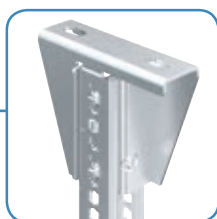
KOPPLAAT PFR41S: EENVOUDIG ZONDER SCHROEVEN HET PROFIEL BEVESTIGEN AAN DE KOPPLAAT
